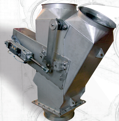
2-Wege-Verteiler 2-way-distributor from square to round Distributeur 2 voies
